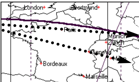
Le trajet de l'éclipse du 11 août et celui des tempêtes du 26 au 28 décembre.
